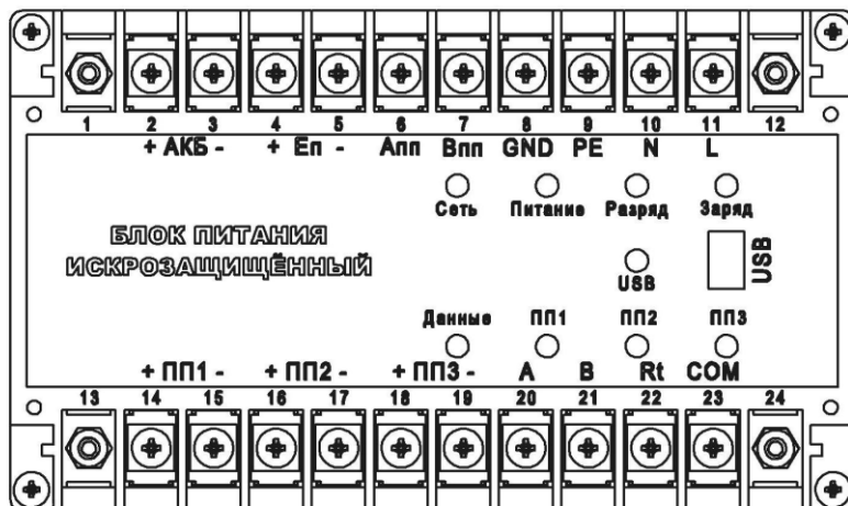
Рисунок В.2– Лицевая панель БПИ с USB разъемом
